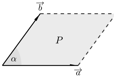
Slika 5.4: Paralelogram razapet vektorima \vec{a} i \vec{b}
