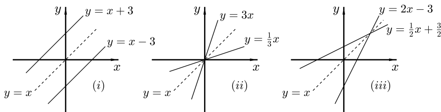
Slika 9.6: Primjer 9.4
