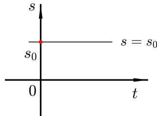
Slika 8.11: s - t dijagram - prikaz mirovanja
