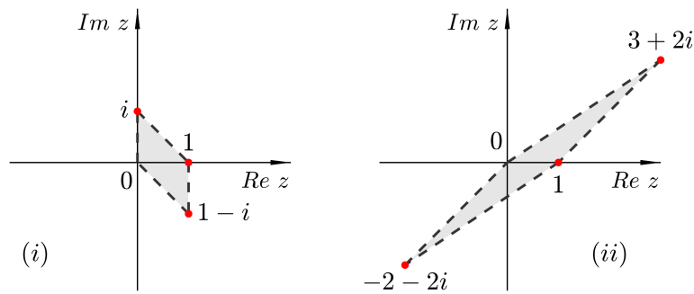
Slika 1.11: Primjer 1.4
