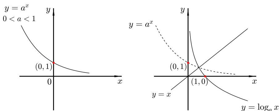
Slika 9.14: Grafovi eksponencijalne i logaritamske funkcije s bazom a manjom od 1
