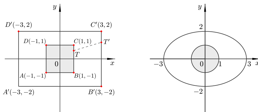
Slika 7.5: Primjer 7.1 (iv)
