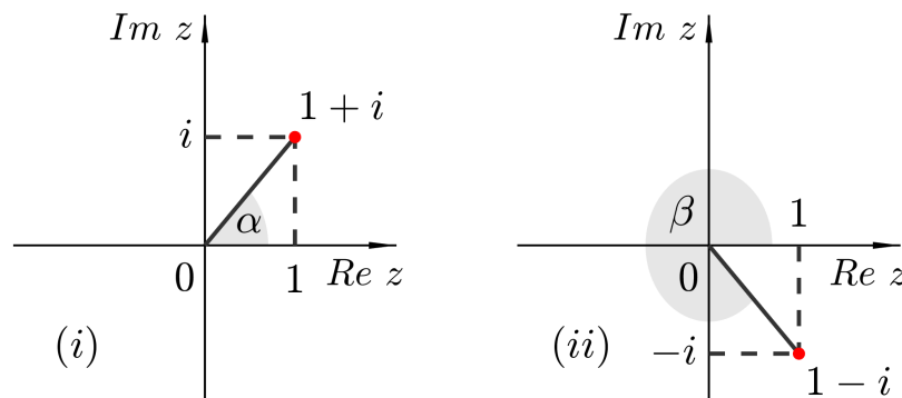
Slika 1.13: Primjer 1.5
