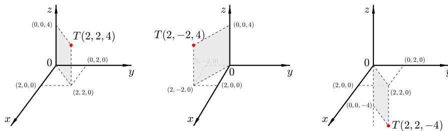
Slika 2.13: Primjer 2.2
