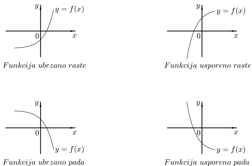
Slika 8.10: Ubrzani rast/pad i usporeni rast/pad
