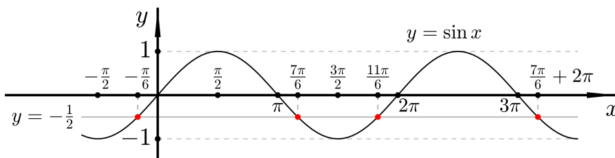
Slika 9.27: Primjer 9.13
