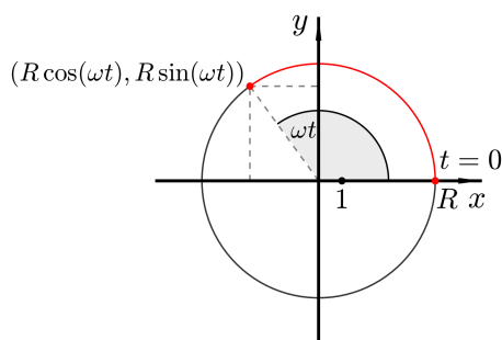
Slika 9.20: Primjer 9.10
