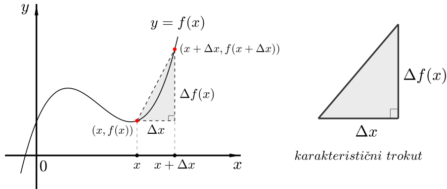
Slika 10.2: Karakteristični trokut
