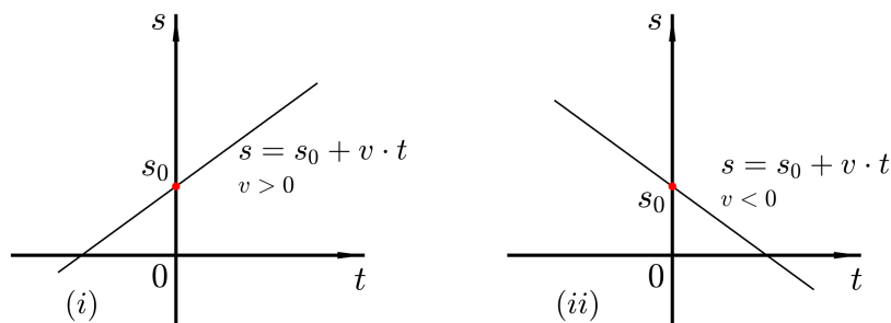
Slika 8.12: s - t dijagram - prikaz jednolikog gibanja
