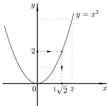
Slika 9.10: Primjer 9.5
