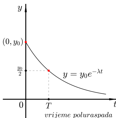
Slika 9.15: Primjer 9.7
