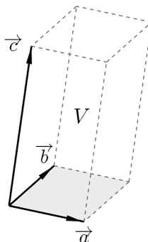
Slika 5.6: Paralelepiped razapet vektorima \vec{a} , \vec{b} i \vec{c}
