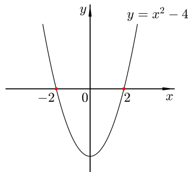
Slika 8.6: Primjer 8.8
