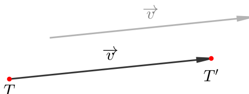
Slika 3.1: Translacija
