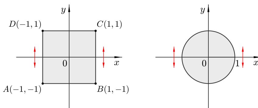
Slika 7.1: Primjer 7.1 (i)
