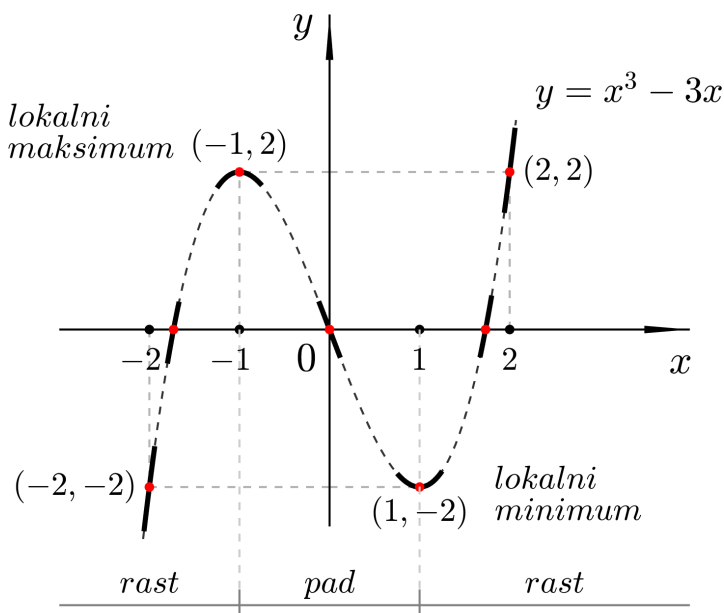
Slika 13.10: Primjer 13.1
