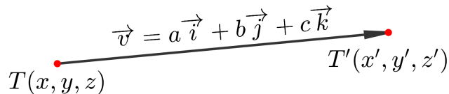
Slika 3.6: Translacija prostora
