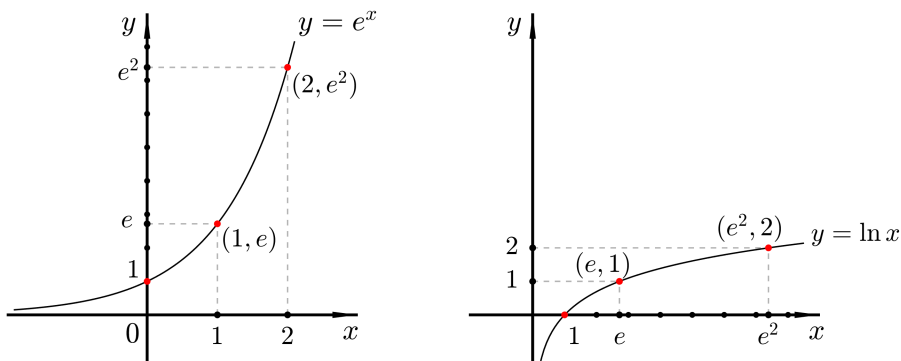
Slika 9.13: Primjer 9.6
