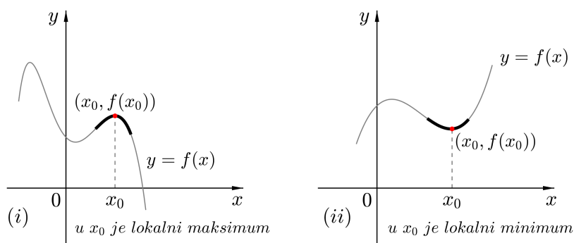
Slika 13.2: Točka lokalnog maksimuma, odnosno minimuma funkcije
