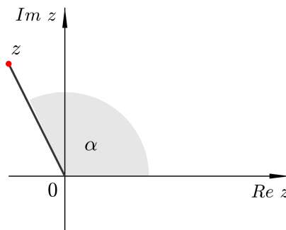
Slika 1.14: Zraka kompleksnih brojeva istog argumenta
