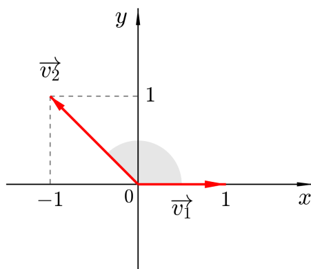
Slika 7.8: Primjer 7.4 (ii)
