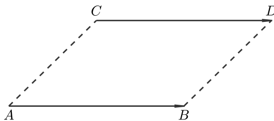
Slika 2.2: Jednakost vektora \overrightarrow{AB} = \overrightarrow{CD}
