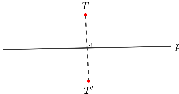
Slika 3.4: Osna simetrija
