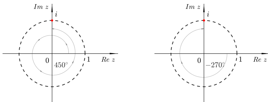
Slika 1.20: Primjer 1.9(i)
