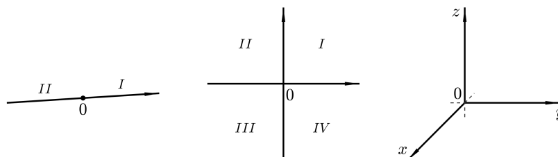
Slika 2.11: Koordinatni polupravci, kvadranti i oktanti
