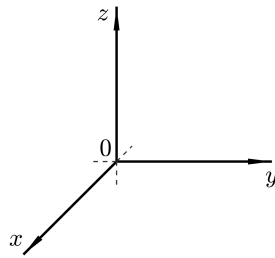
Slika 2.9: Koordinatni prostor
