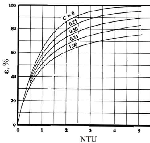
križni izmjenjivač sa oba nemiješana fluida
