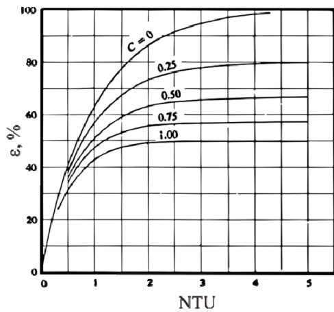
jednostruki istostrujni
