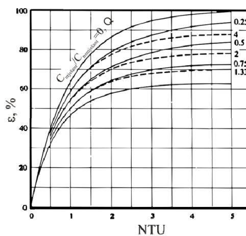
križni izmjenjivač sa jednim miješanim fluidom
