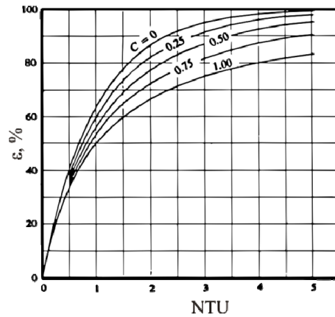
jednostruki protustrujni
