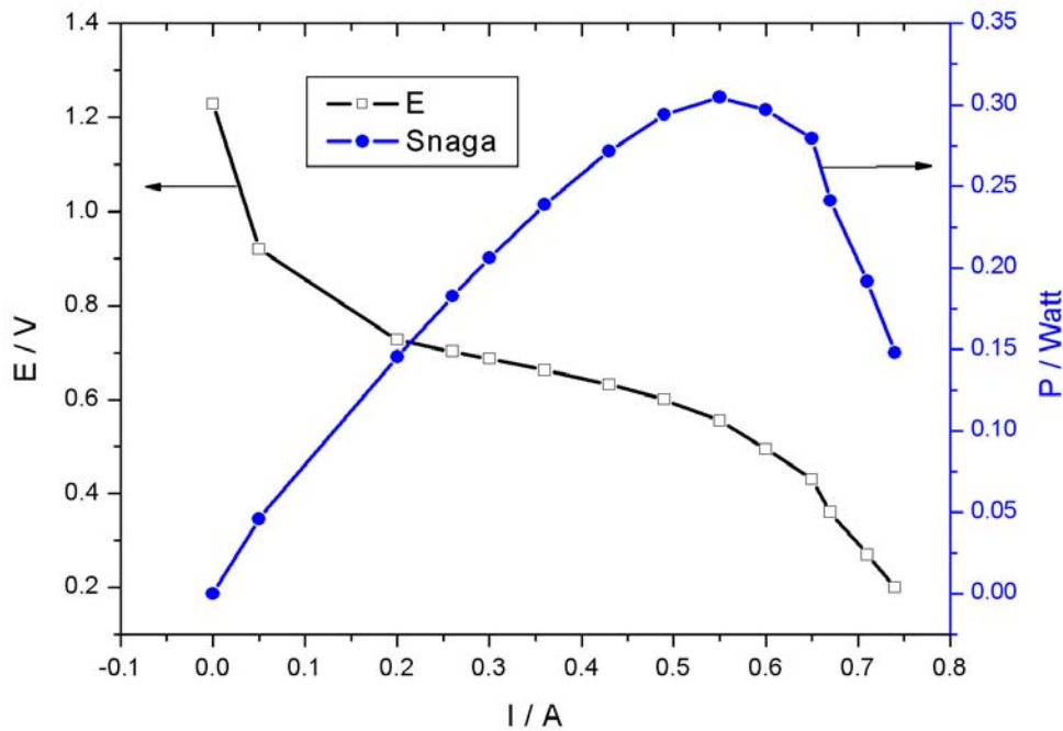
Slika 2. Strujno-naponska karakteristika gorivnog članka i ovisnost snage gorivnog članka o opterećenju
